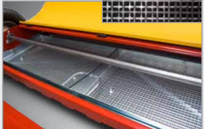
Regulowana średnica oczek sita wibracyjnego 4-10 mm
